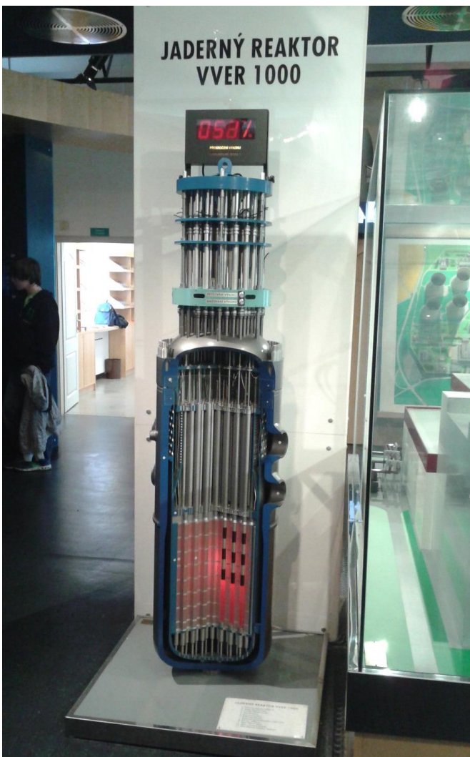
Model jaderného reaktoru
